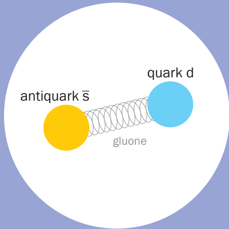
mesone K^0
