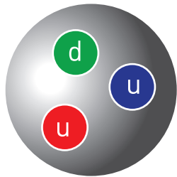
barione
