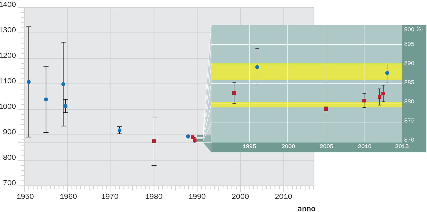
vita media del neutrone (s)
