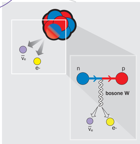
decadimento beta
