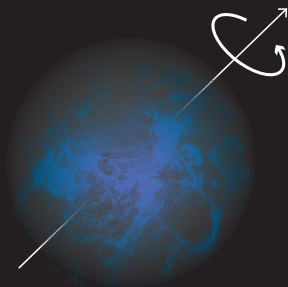
nebulosa in rotazione
