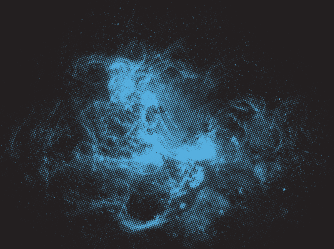
nubi di gas e polveri
