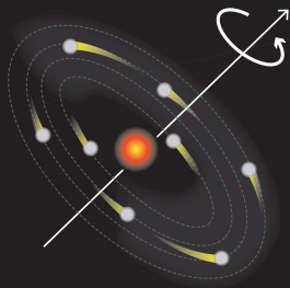
protosole
