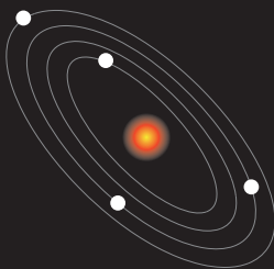
sistema planetario
