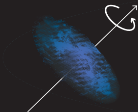
collasso gravitazionale e appiattimento
