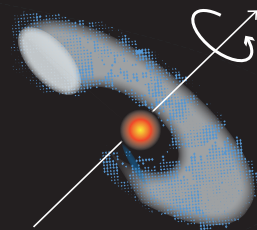
nebulosa solare
